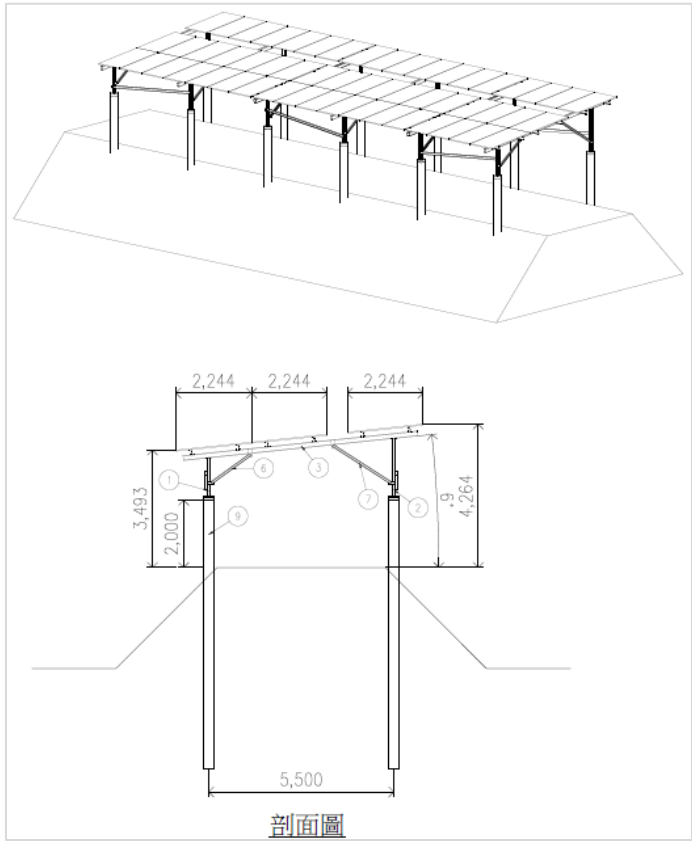
塼堤設置結構
