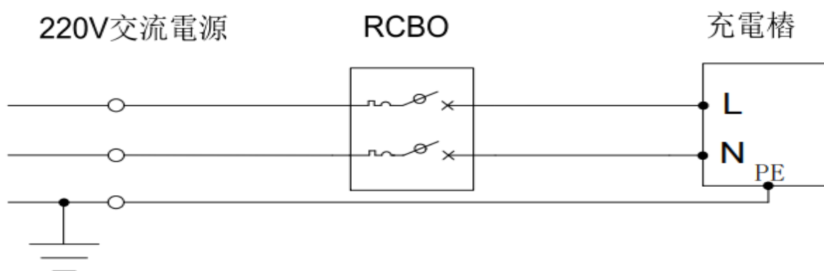
圖 3.1.3.3 電氣系統
