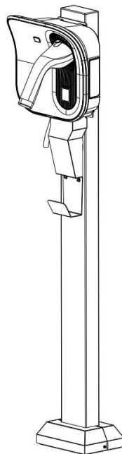
圖 3.2.2.2 ( 6 ) 安裝完成
