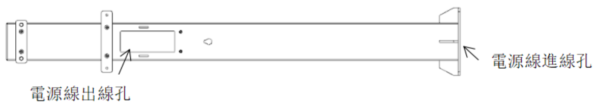
圖 3.2.2.2 ( 2 ) 立柱穿線
