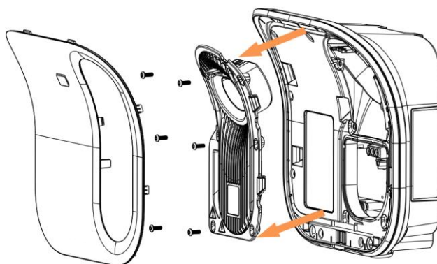
圖 3.2.2.1（6）拆插槍座
