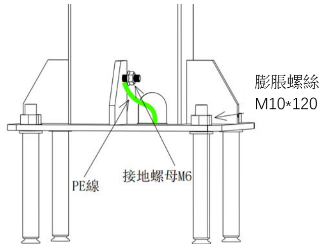
圖 3.2.2.2 ( 3 ) 立柱接地
