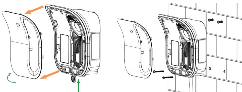
圖 3.2.2.1（5）安裝牆盒
