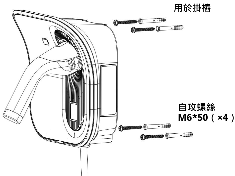
圖 3.2.2.1 ( 1 ) 壁掛式充電樁總裝圖
