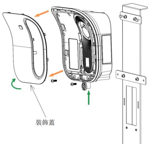
圖 3.2.2.2 ( 4 ) 安裝充電樁
