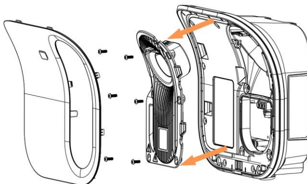
圖 3.2.2.1（6）拆插槍座
