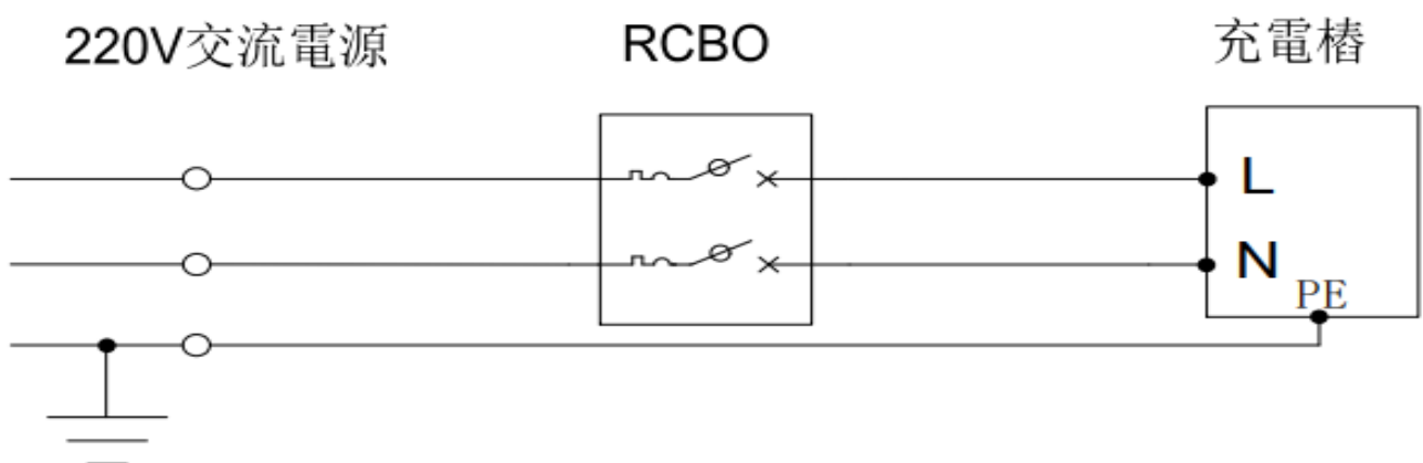
圖 3.1.3.3 電氣系統
