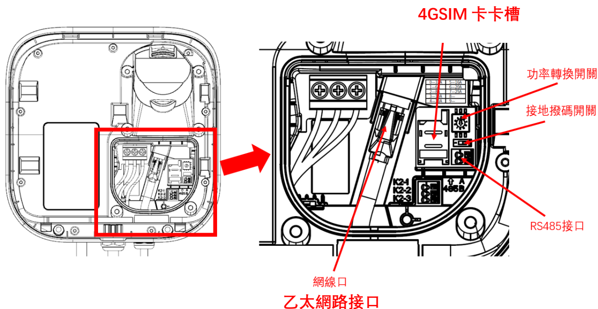
圖 3.2.2.1（8） 乙太網路線
