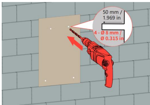
圖 3.2.2.1（3）標記安裝孔
