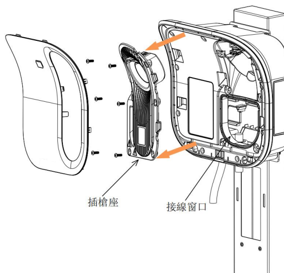
圖 3.2.2.2 ( 5 ) 樁體接線
